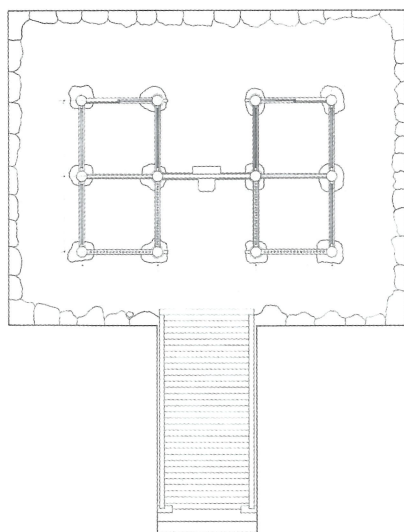
初重平面図
