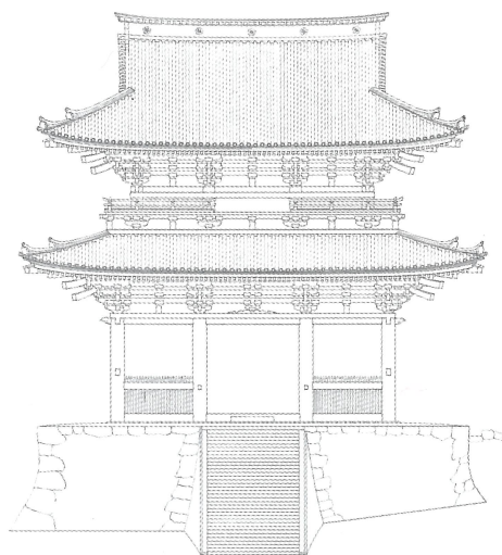
北立面図
