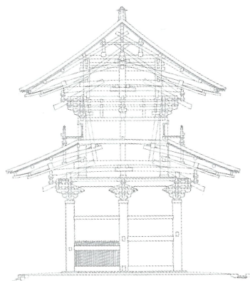
梁行断面図
