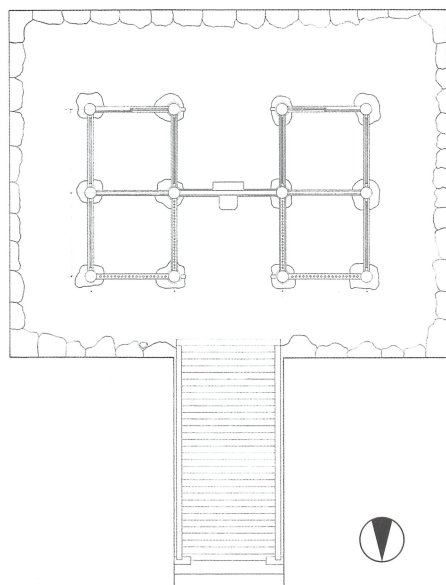
初重平面図
