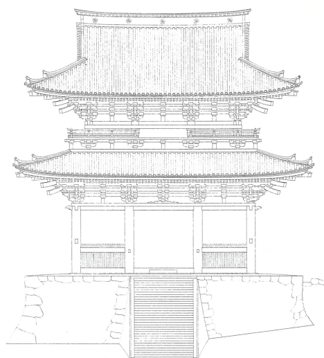
北立面図
